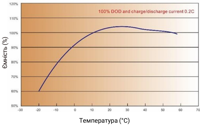
Характеристики заряду/розряду
